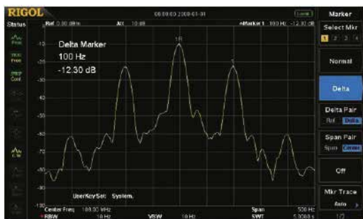
Различие двух соседних частот при RBW 10 Гц
